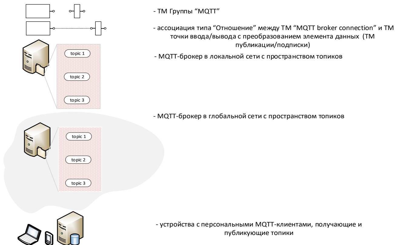
Рисунок 3.2.2 (Обозначения)
