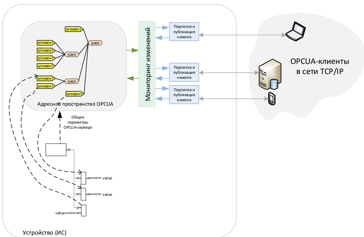
Рисунок 3.5.1 (Типовая схема сервера)
