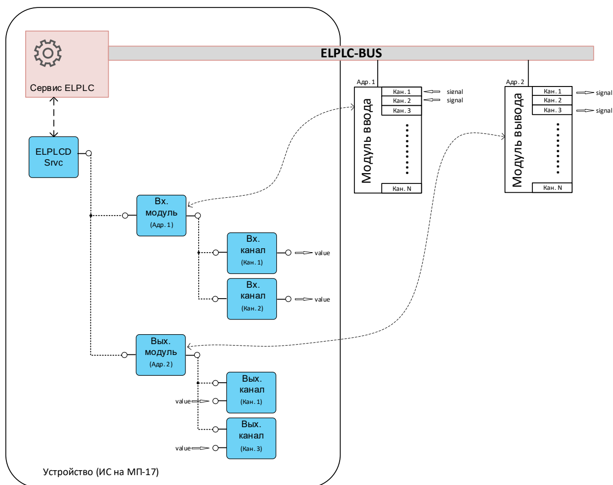
Рисунок 3.6.1 (Общая схема)
