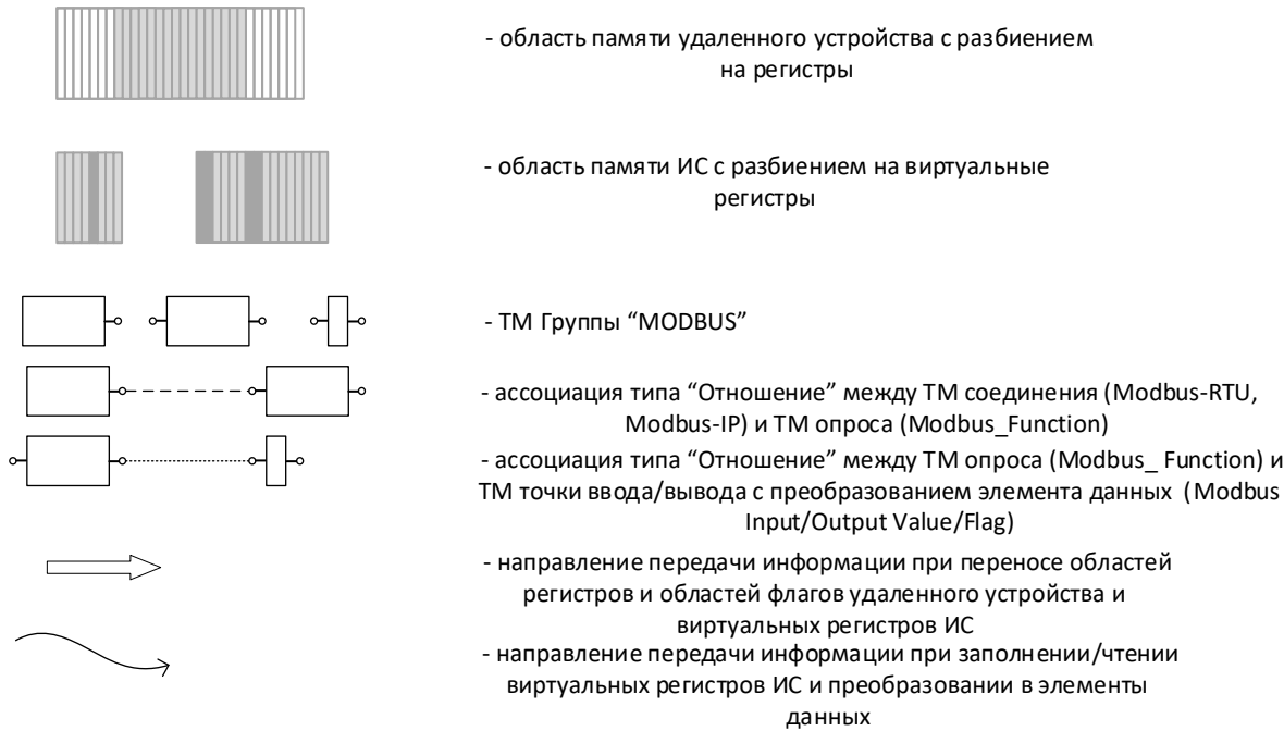
Рисунок 3.1.3 (Обозначения)
